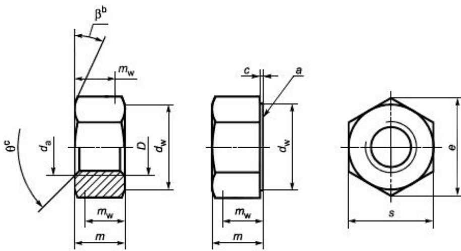
Рисунок 1. Размеры гаек
